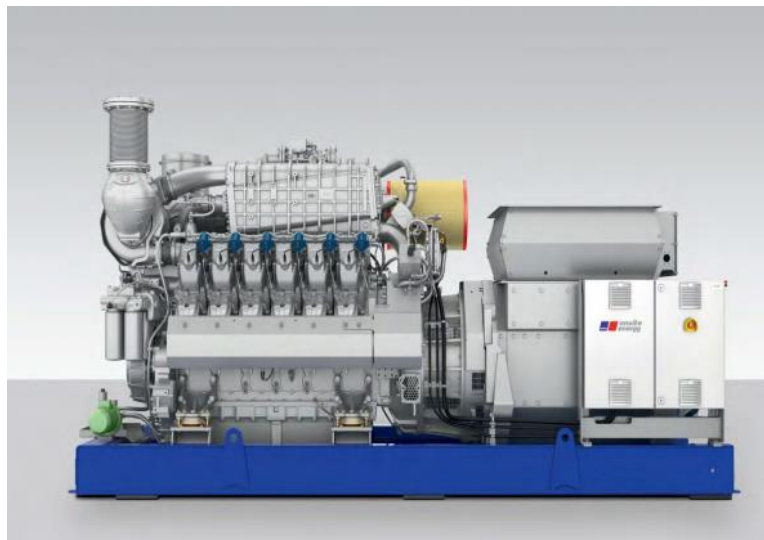
Figura 2-3 immagini fotografiche di un impianto analogo.
