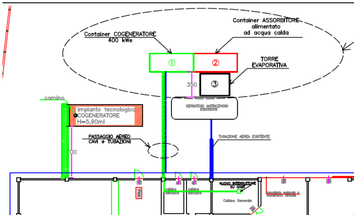
Figura 2-4 Schema della disposizione dell'impianto.
