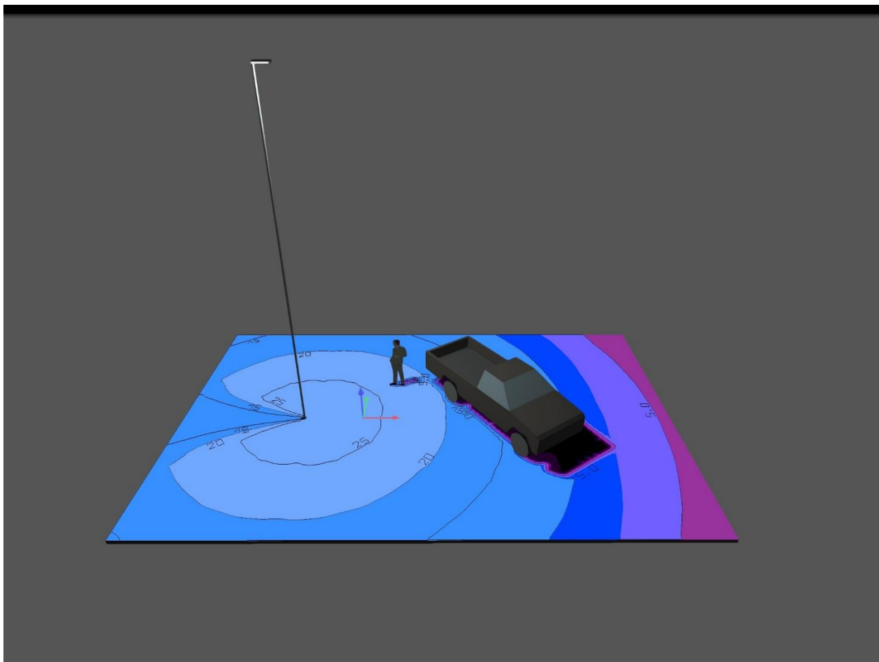
Diagramma di esempio per l'illuminazione di un'area 15x10 mt
