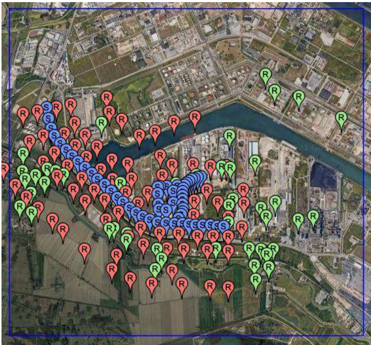
Immagine n. 9 - Azzurro l'asse stradale - Rosso i Recettori stradali - Verde i Recettori discreti - estratta da software MMS Caline
