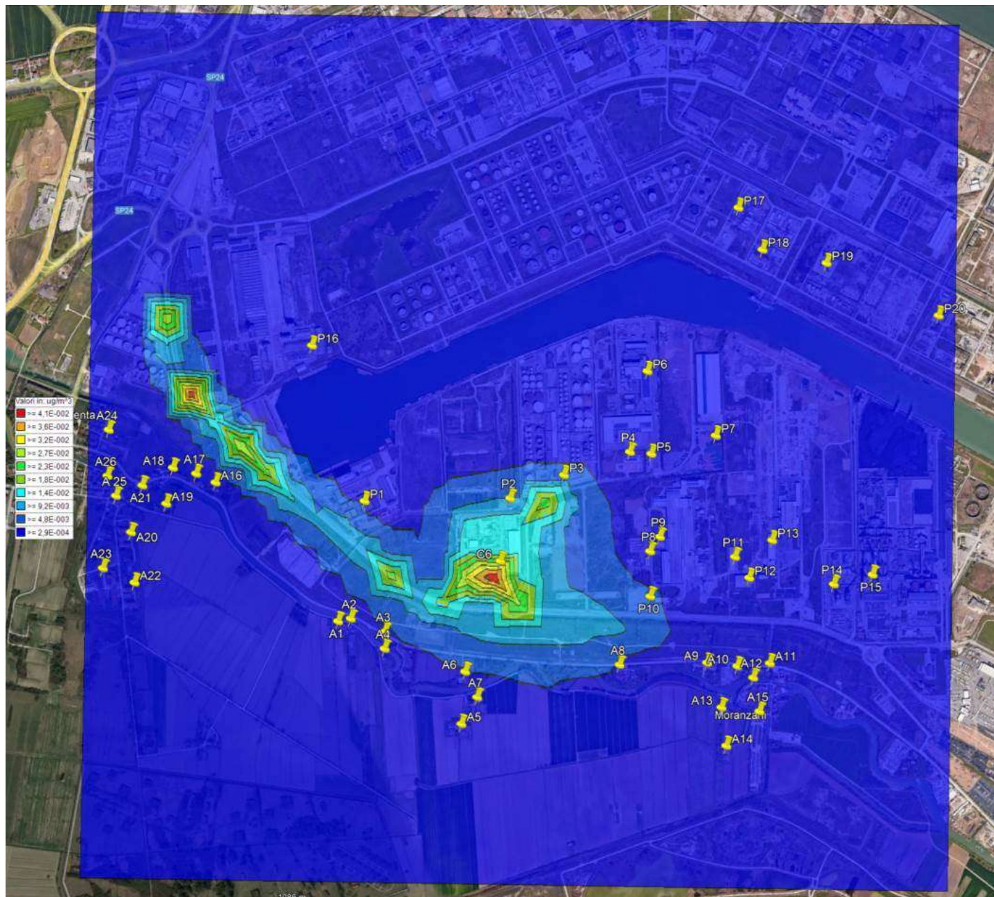
Immagine n. 35 - 99,79° percentile \text{NO}_2
