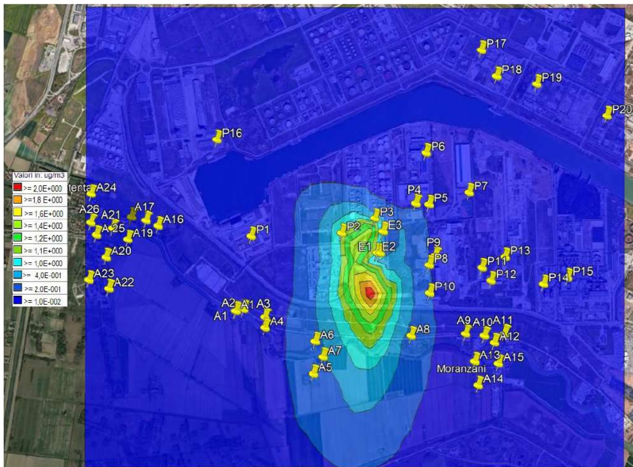
Immagine n. 26 – PM10 90,41° percentile
