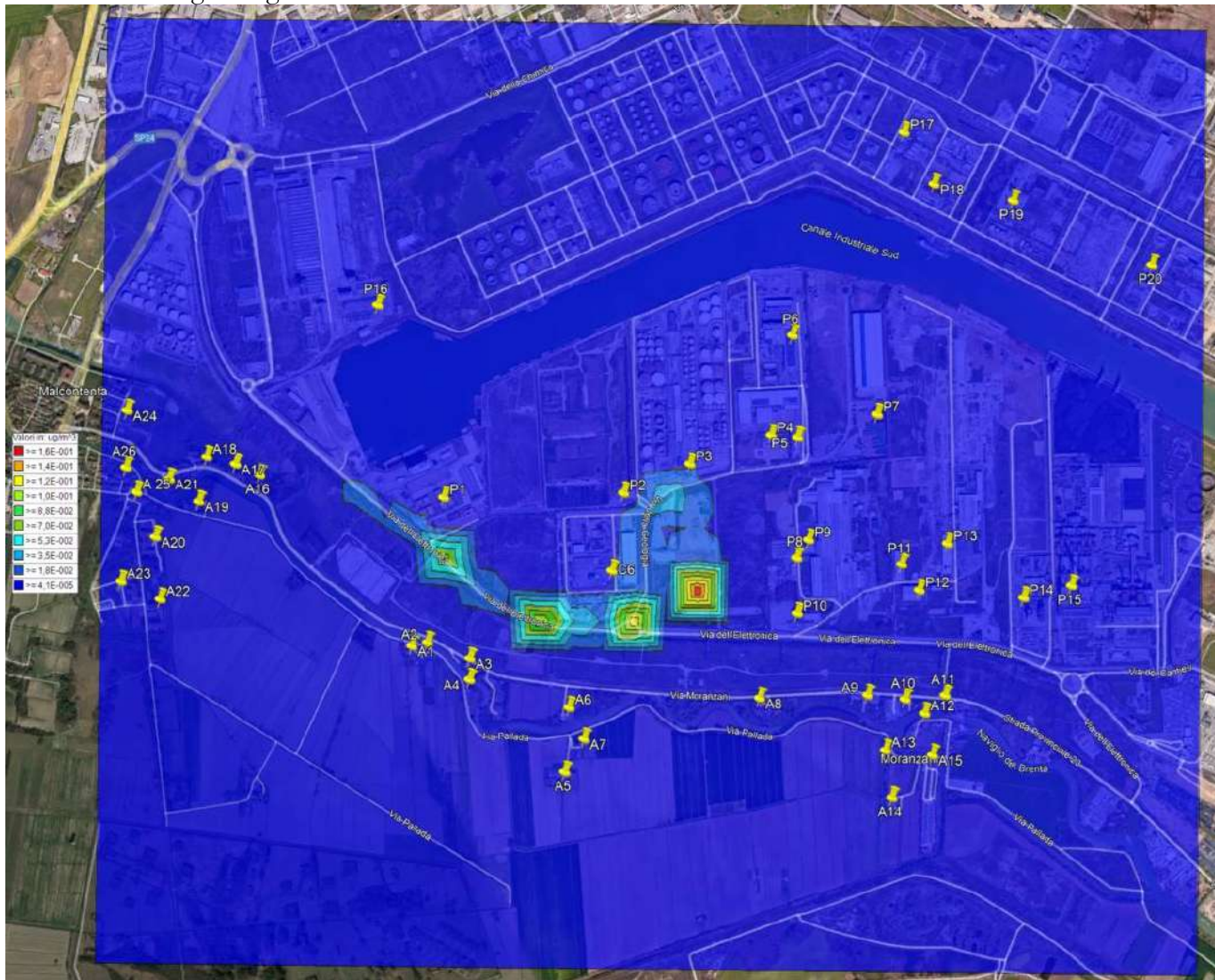
Immagine n. 44 – concentrazioni medie annuali \text{NO}_2
