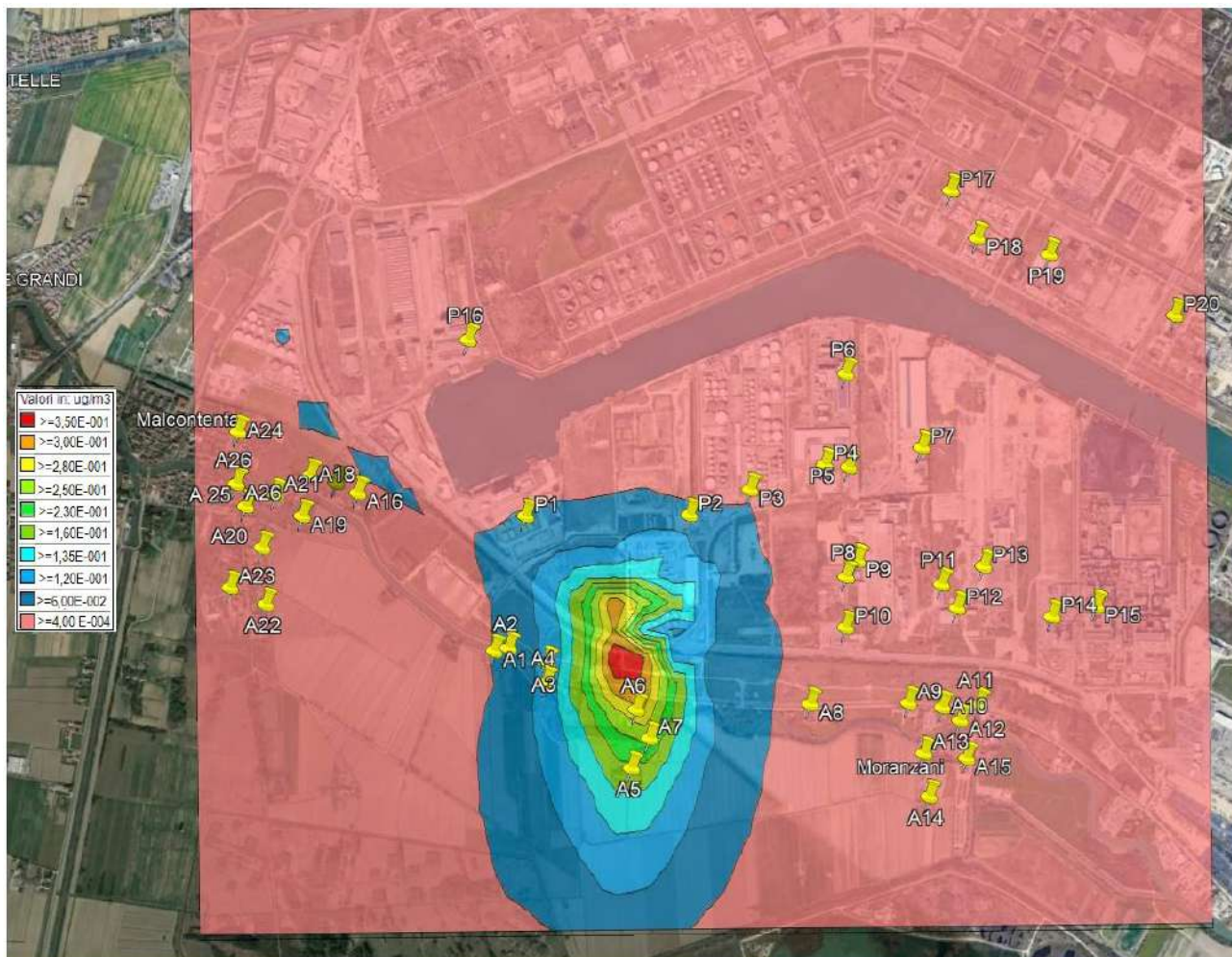
Immagine n. 20 - PM 10 complessive- 90,41° percentile
