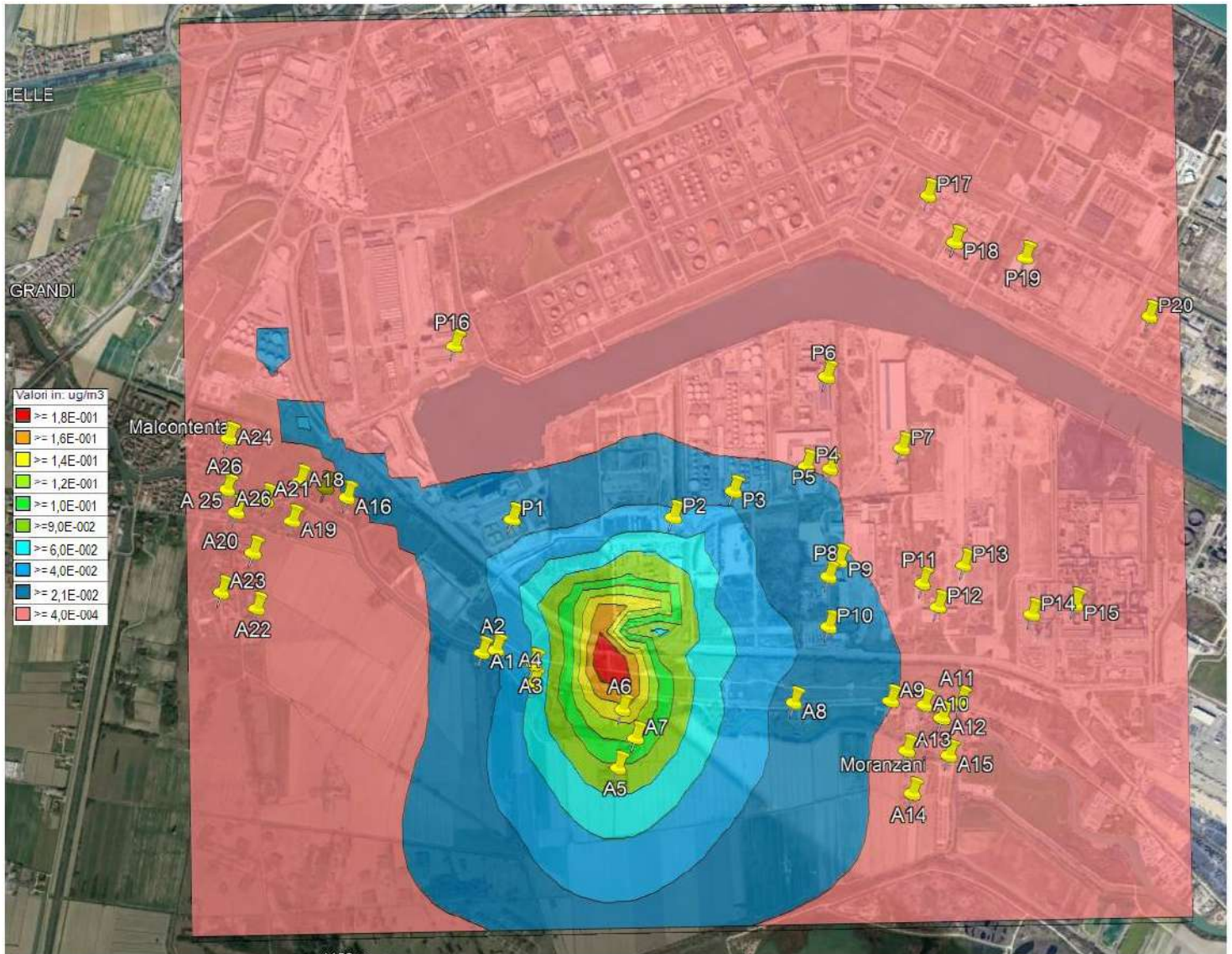
Immagine n. 19 - PM 10 complessive- valori medi
