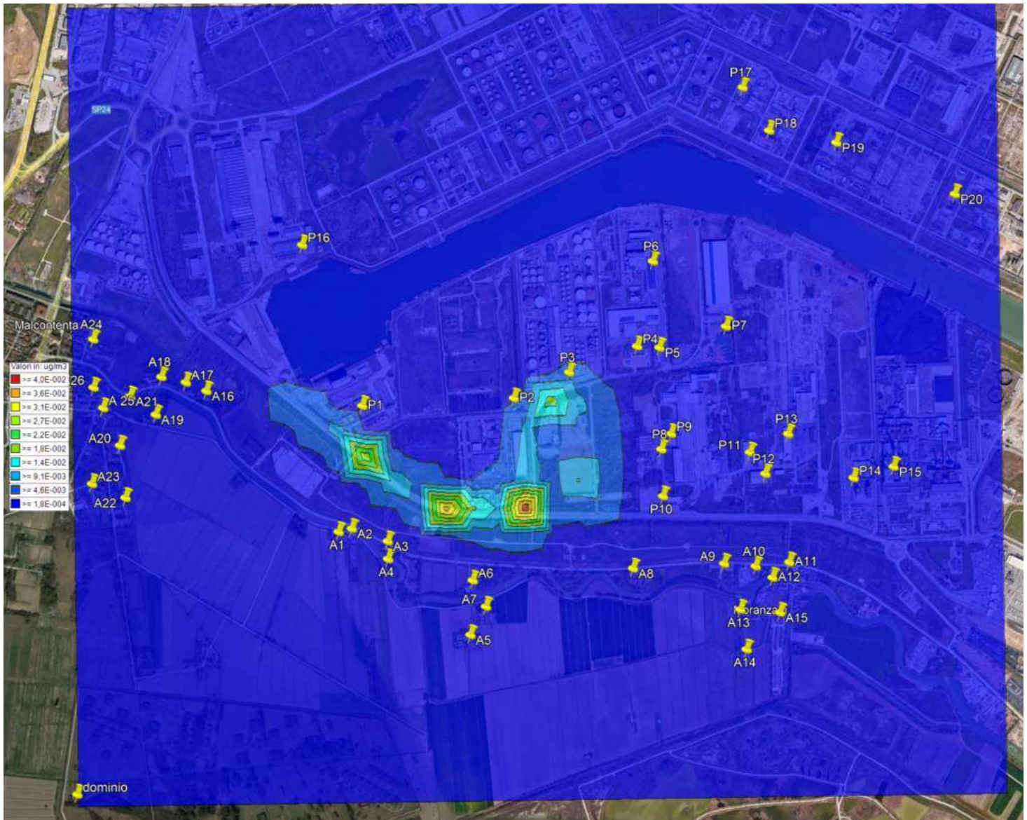
Immagine n. 40 – concentrazioni PM 10 medio annuo
