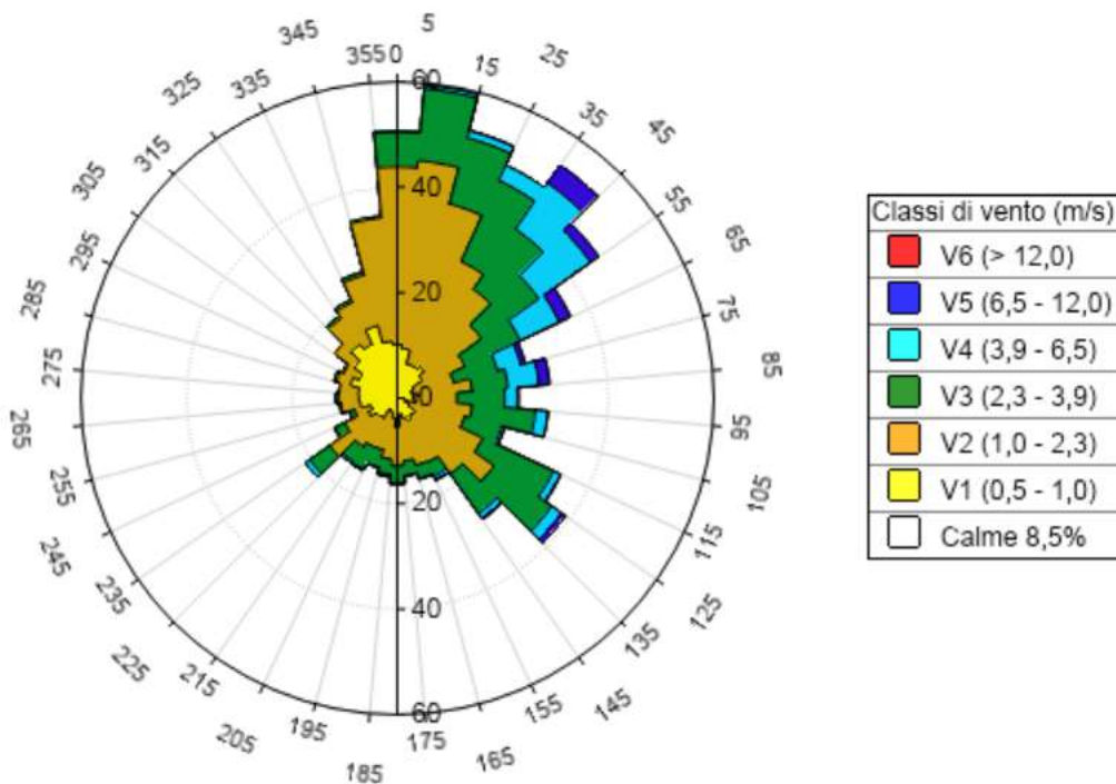
Rosa dei venti (velocità del vento in m/s)
