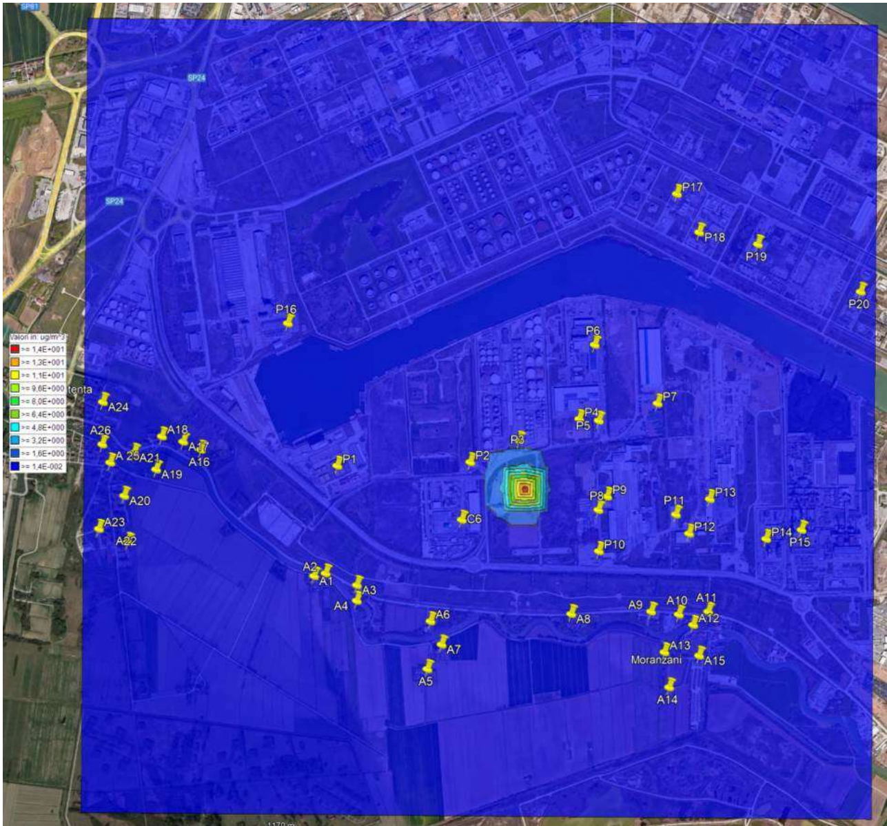
Immagine n. 60 – concentrazioni medie annuali NO 2
