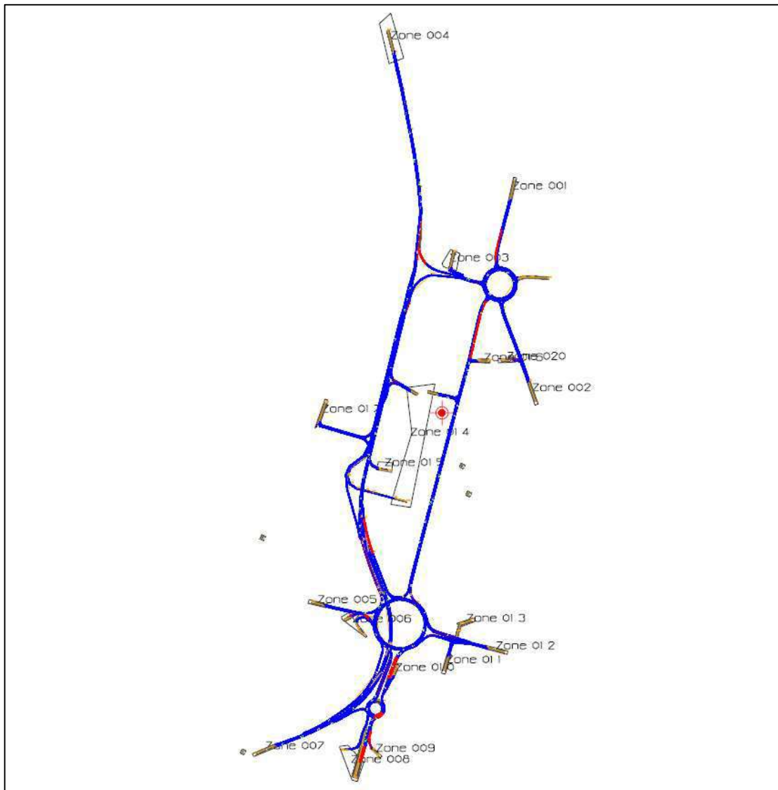
Stato di progetto SDP: Livello di Servizio per ramo (sopra: blu LdS A, rosso LdS peggiore di C)
