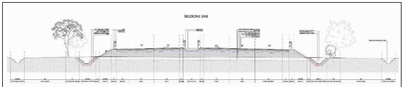
Sezione tipo stradale in rilievo prevista per la “Via del Mare” (da progetto preliminare, 2007)
