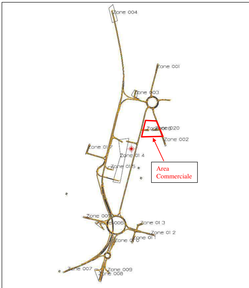
Grafo della rete viaria nello Stato di Progetto
