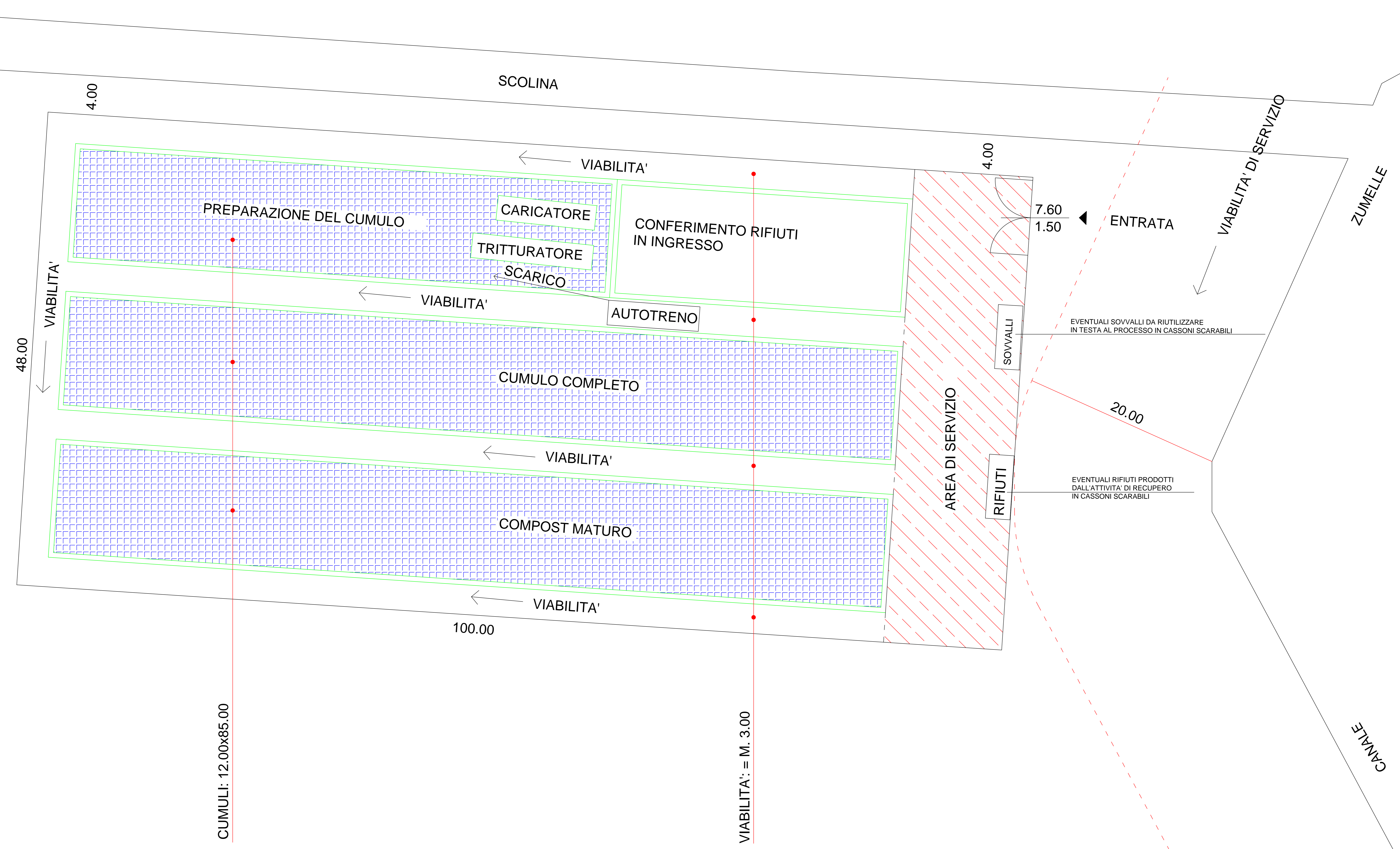
PLANIMETREIA TECNICA
