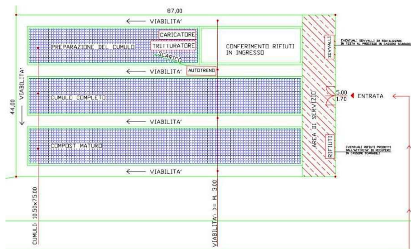
Layout dell'impianto
