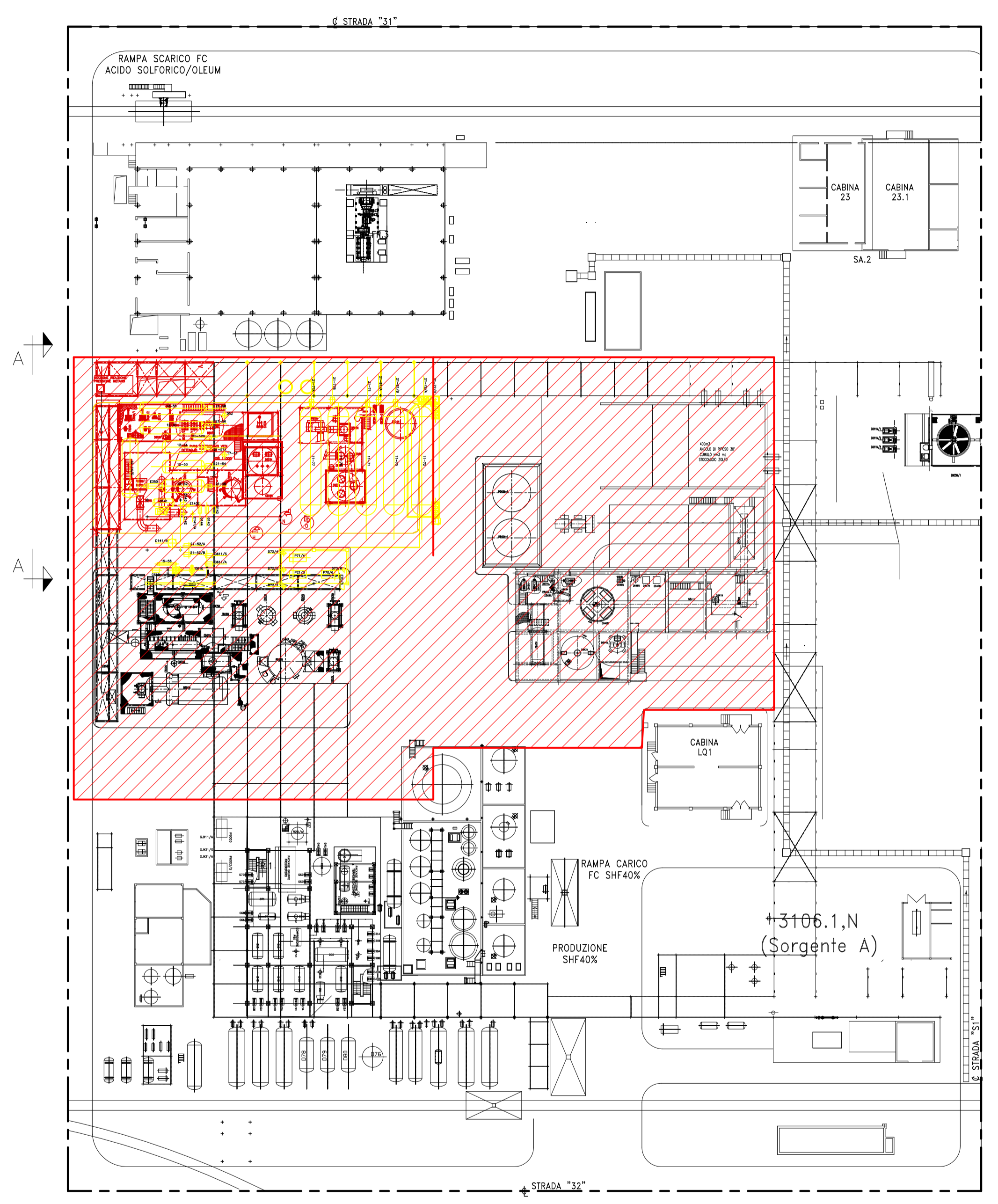
PIANTA SCALA 1:200
