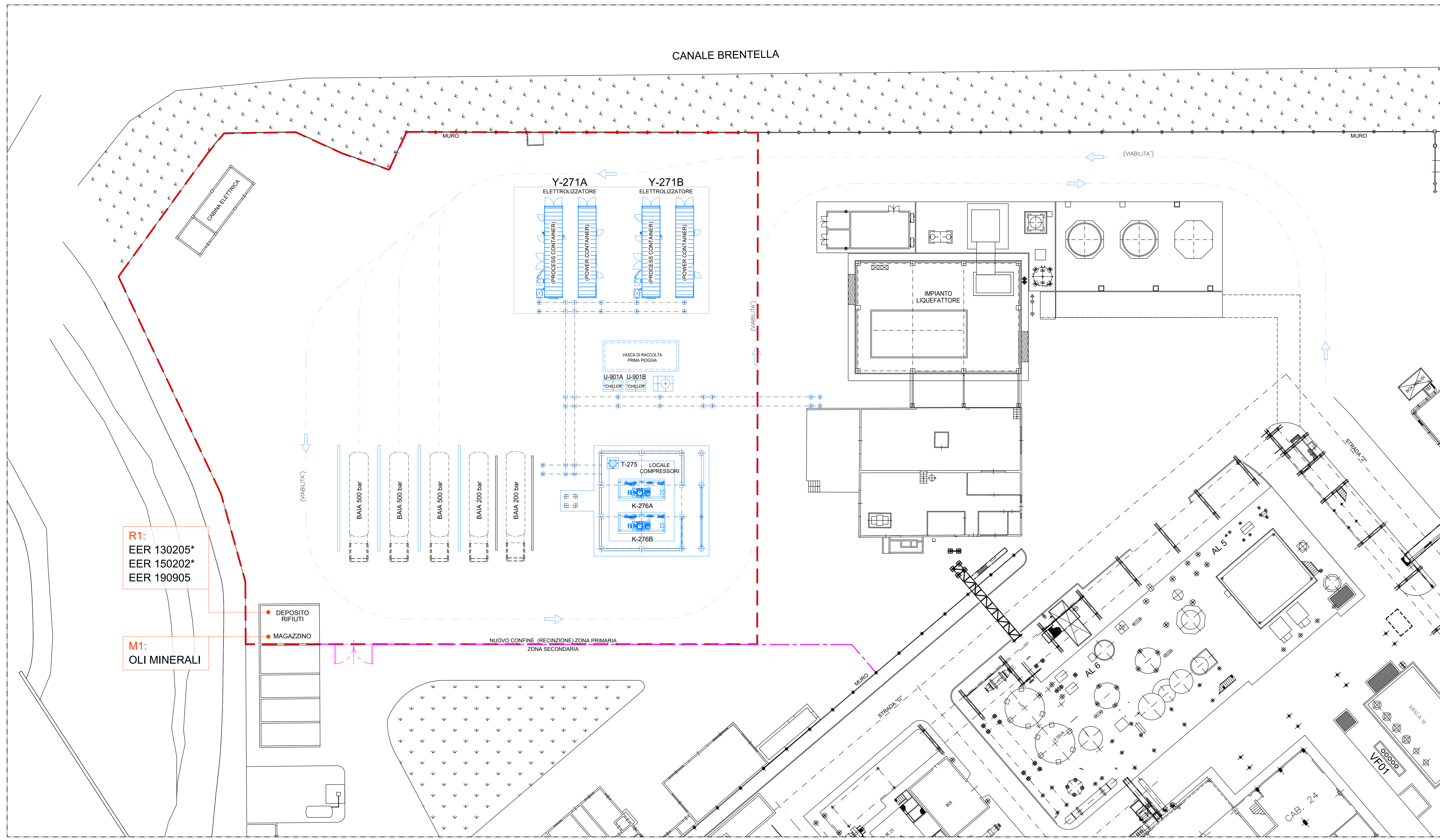
- PIANTA UBICAZIONE -
