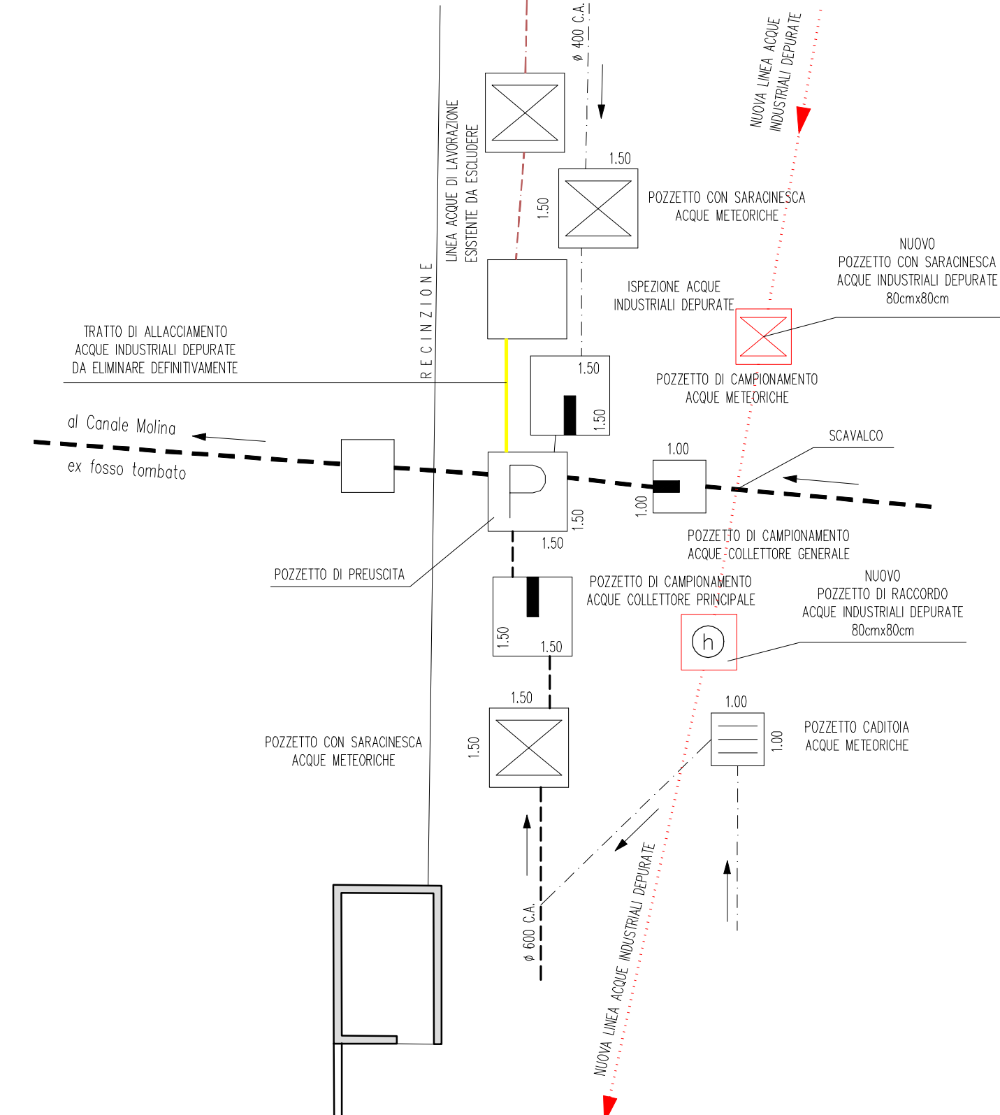
POZZETTI DI PREUSCITA 1:100
