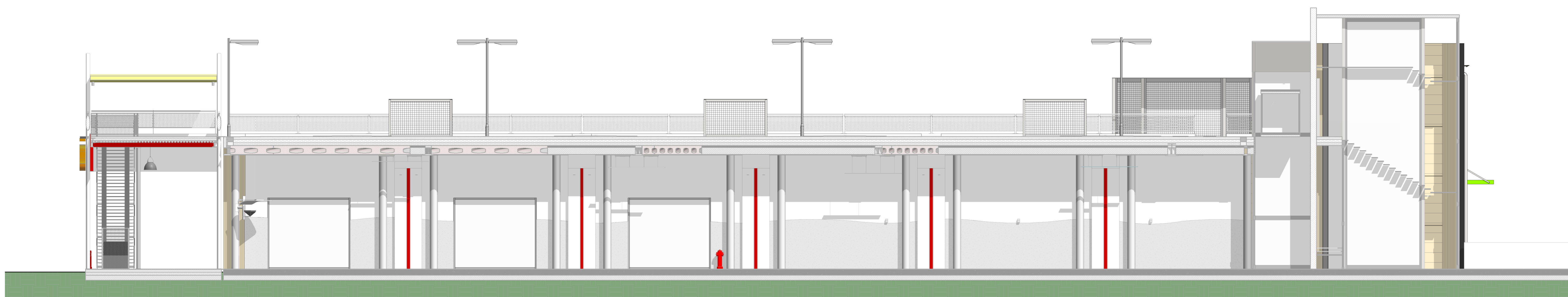
PROSPETTO SUD scala 1 : 100
