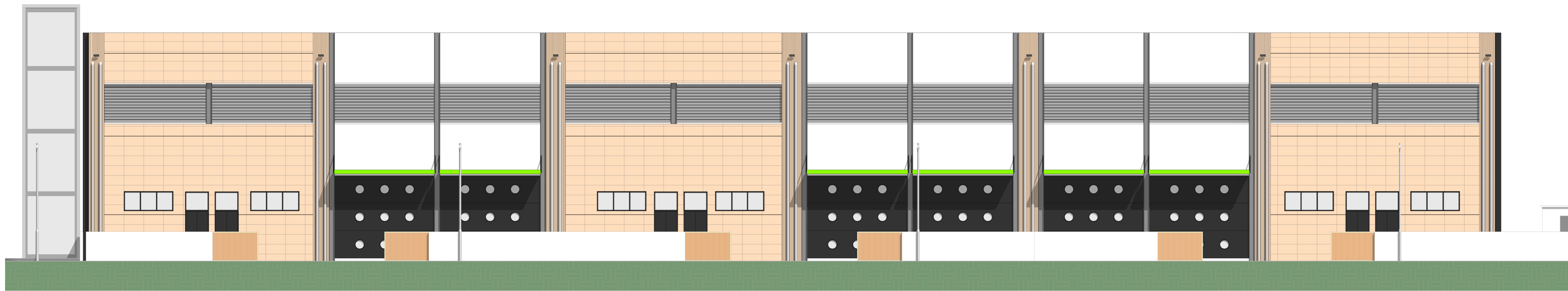
PROSPETTO EST scala 1 : 100
