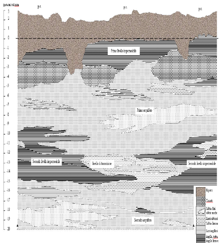
Figura 2.2.5 – Modello idrogeologico locale dell'area di Porto Marghera
