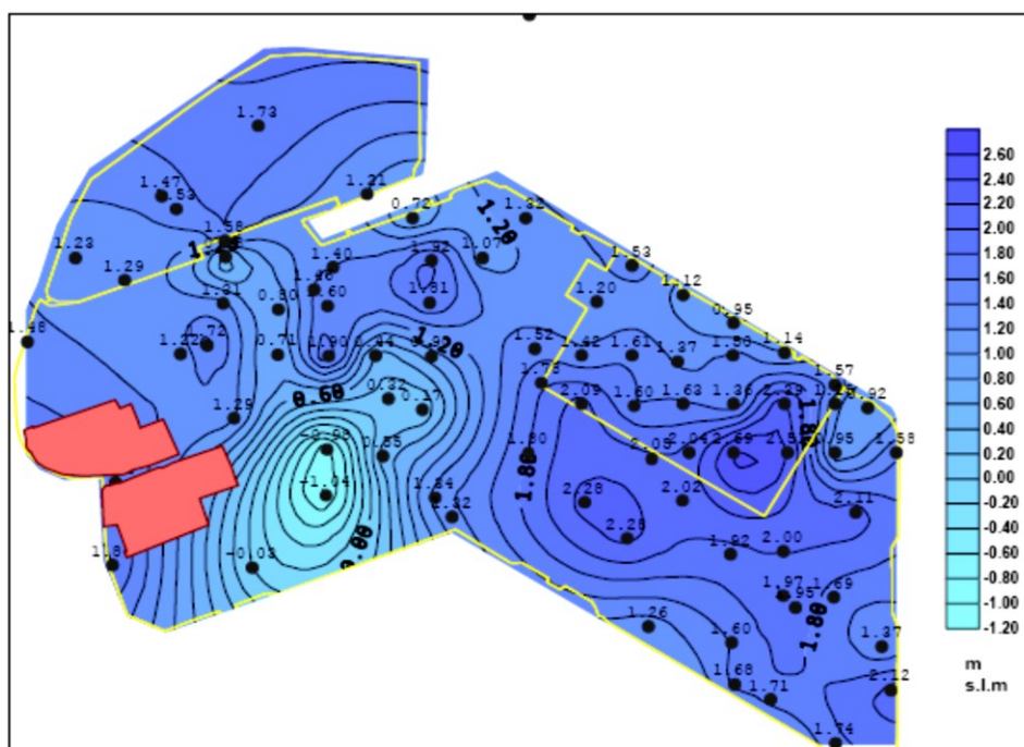
Figura 2.2.4 – Ricostruzione dell’assetto piezometrico dell’acqua nel riporto nella macroarea della chimica (Indagine Idrogeologia Porto Marghera)
