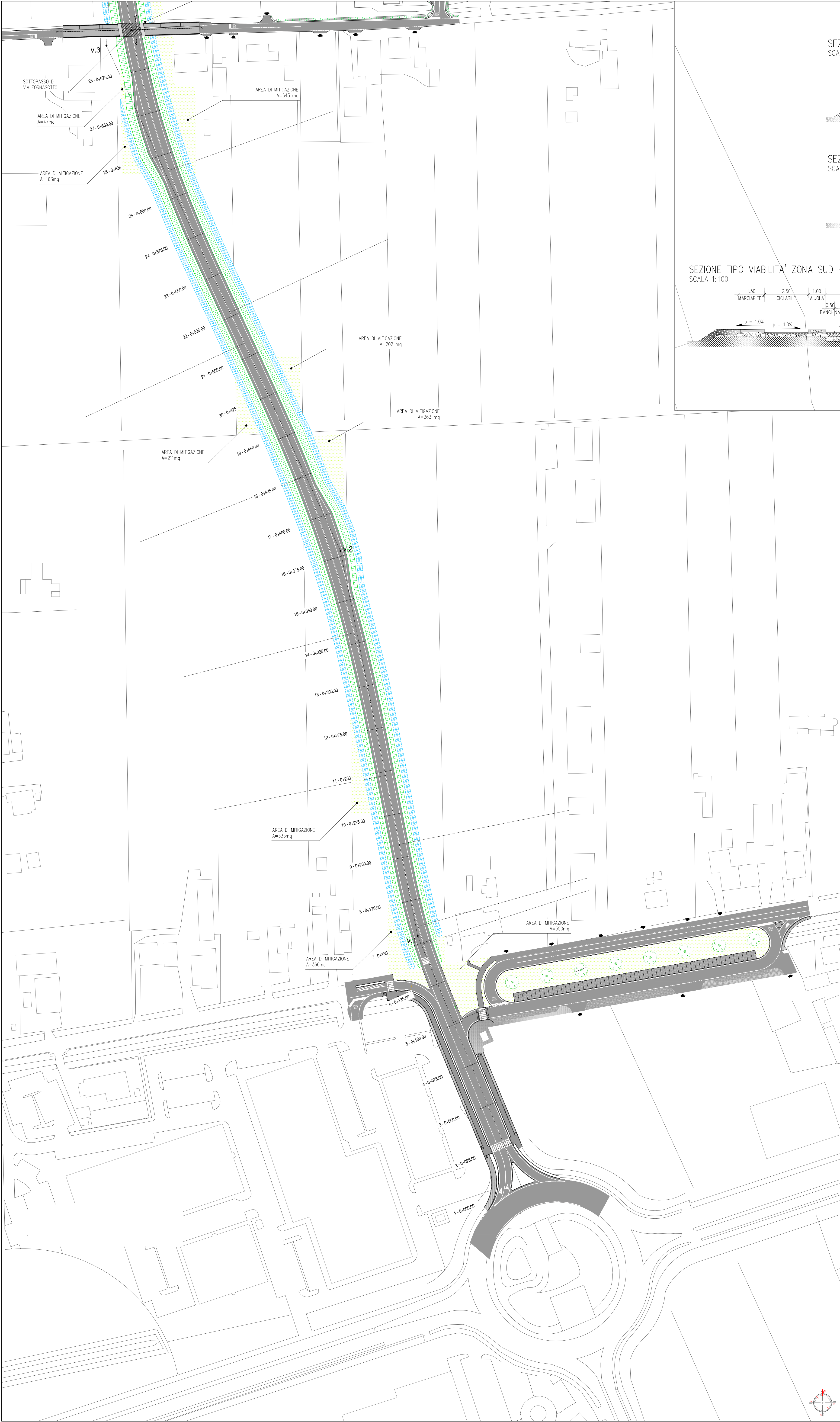
PLANIMETRIA DI PROGETTO – QUADRO 2 | Scala 1:1000
