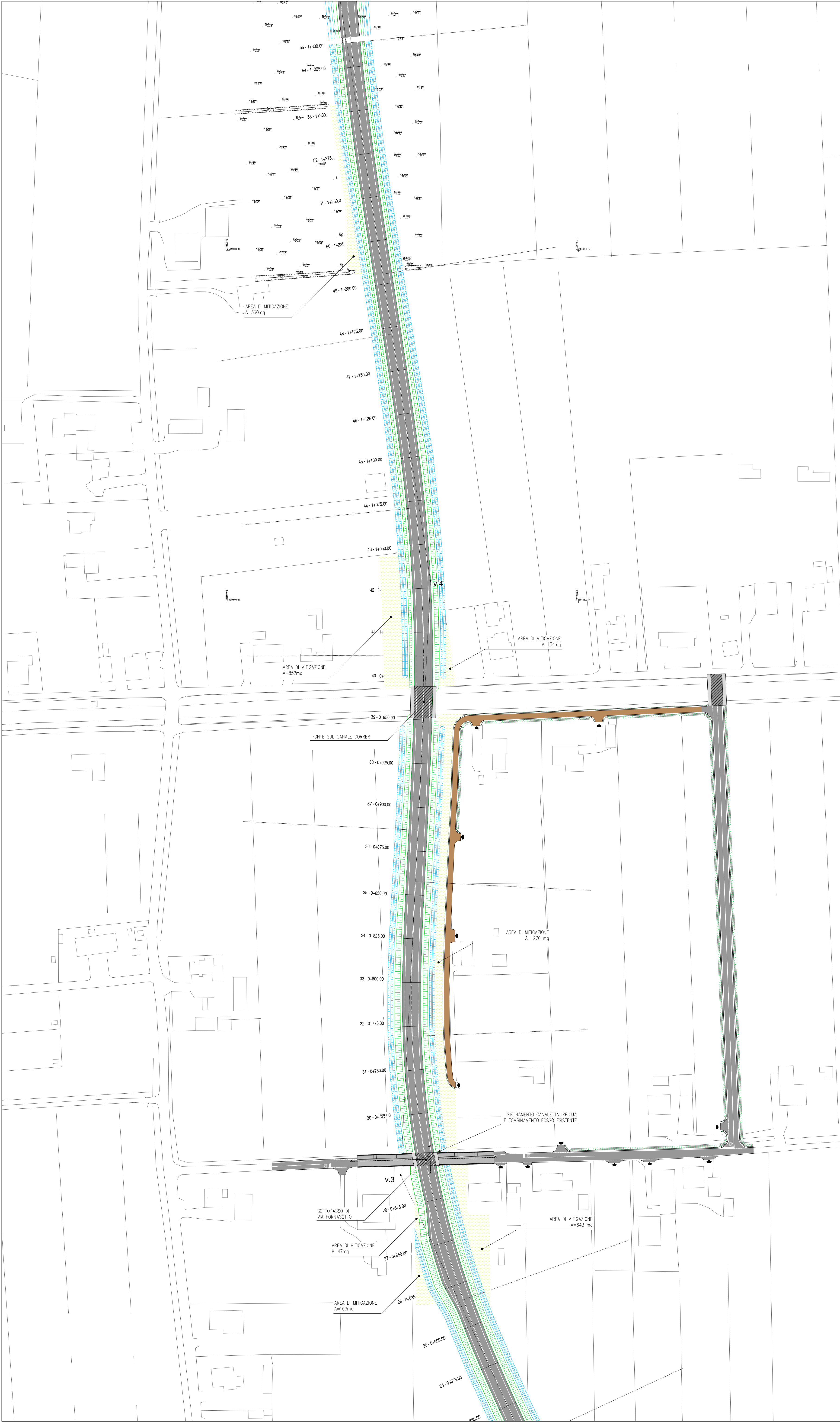
PLANIMETRIA DI PROGETTO – QUADRO 1 | Scala 1:1000
