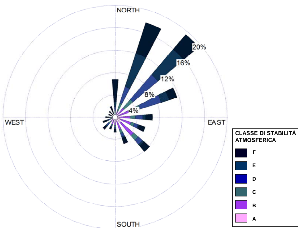
Figura 4.1. Rosa dei venti per le classi di stabilità atmosferica (Marghera, 2011)
