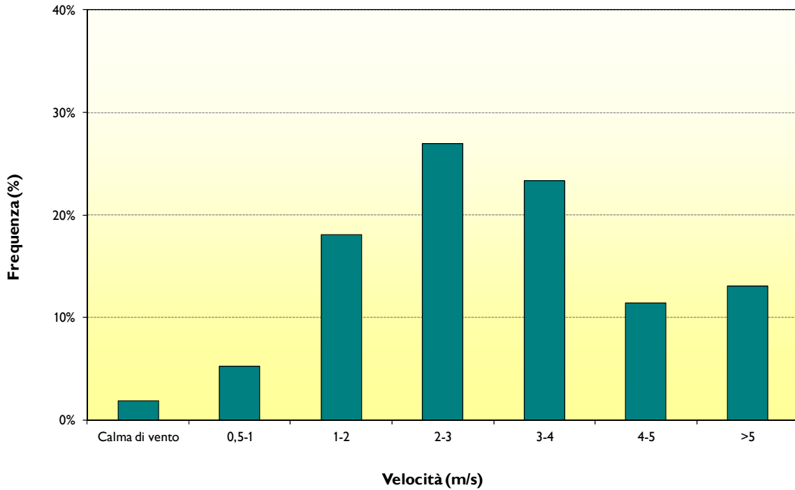
Figura 3.1. Distribuzione annuale di frequenza delle classi di velocità (Marghera, 2011)
