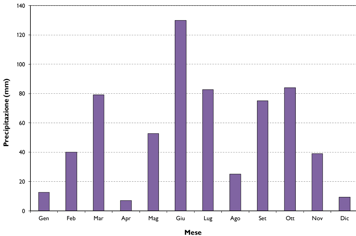
Figura 5.1. Andamento della precipitazione cumulata mensile (Marghera, 2011)
