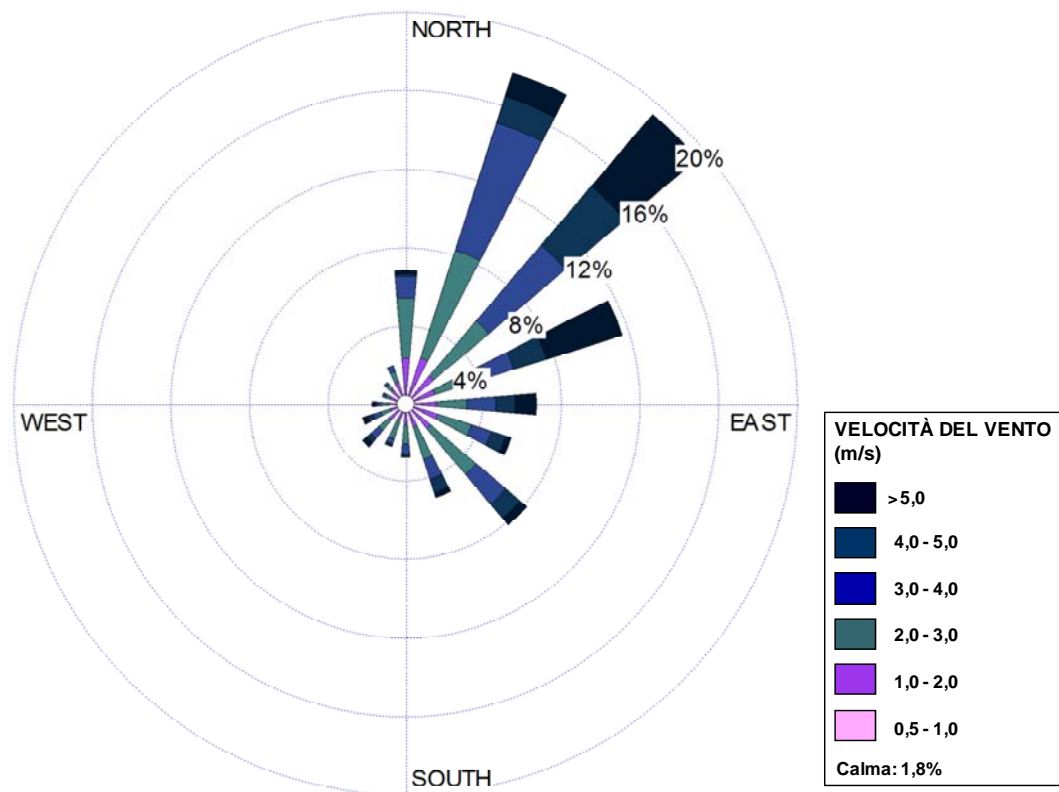
Figura 3.2. Rosa dei venti per le classi di velocità (Marghera, 2011)
