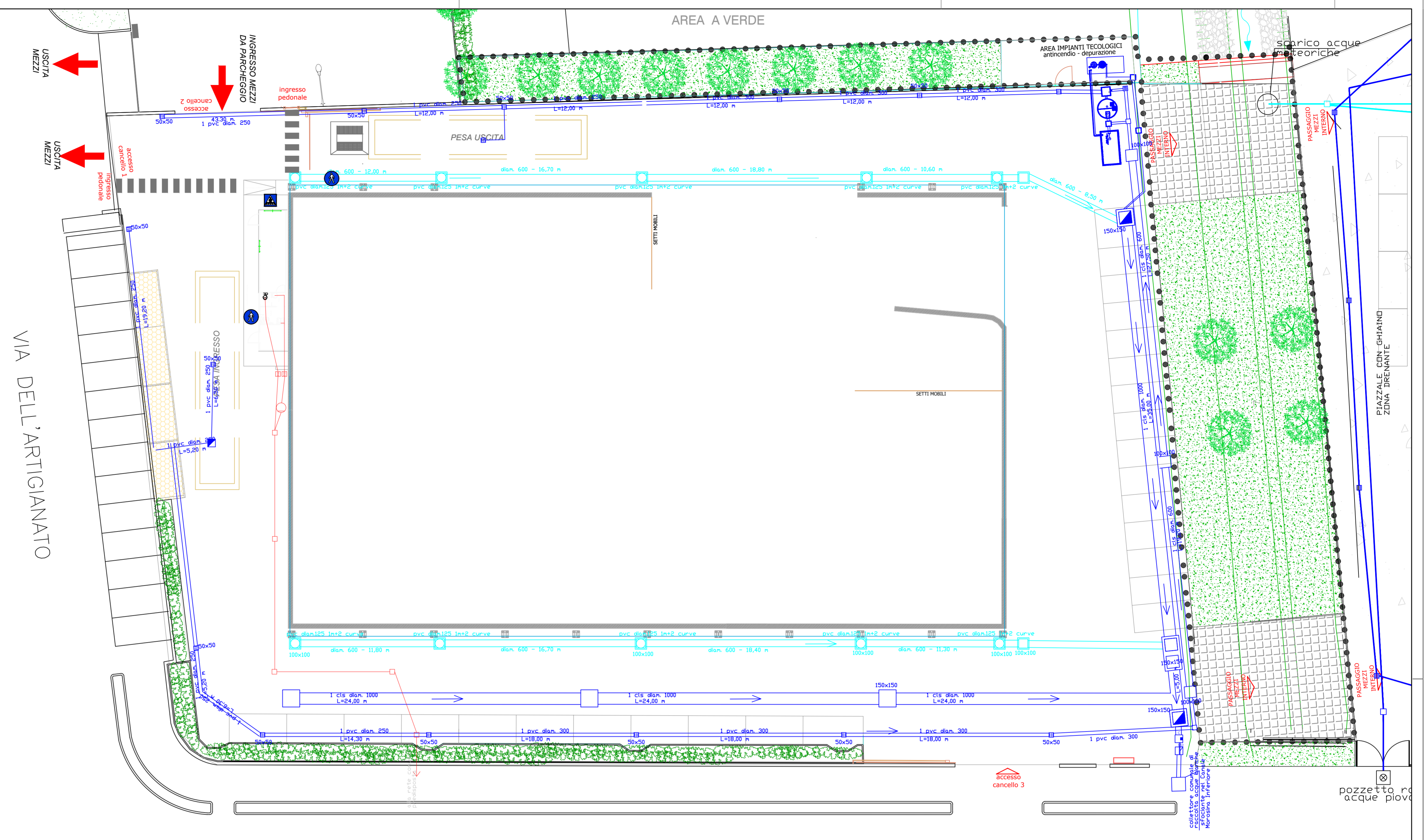
Planimetria reti acque meteoriche e reflue civ. 56 SCALA 1:200
